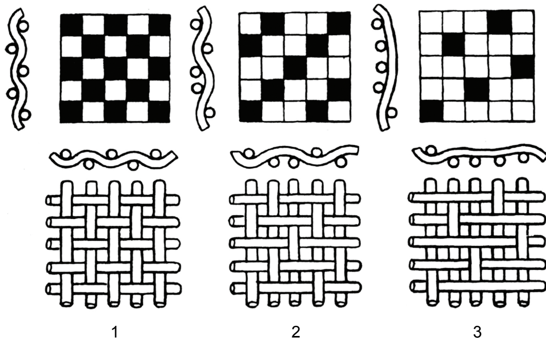
Рис. 2.1. Прості переплетення: 1 – полотняне; 2 – саржеве; 3 – сатинове (атласне)
