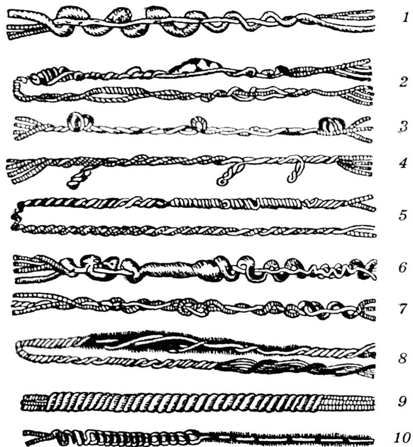
Рис. 1.5. Види пряді фасонного кручення: 1 – спіральна; 2 – вузликова; 3 – петляста; 4 – зі скрутинами; 5 – застилиста; 6 – комбінована; 7 – епонж; 8 – з рівничним ефектом; 9 – із зовнішньою обмоткою; 10 – синель
