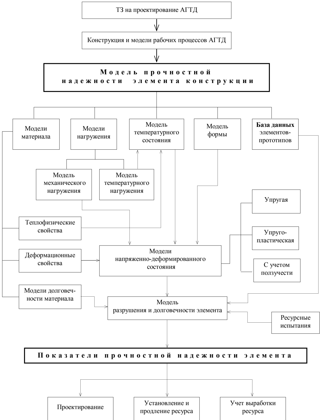
Рис. 1. Структура модели прочностной надежности элемента конструкции АГТД:
