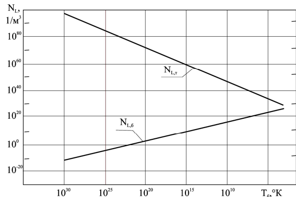
Рис. 6. Влияние температуры T_{\bar{o}} на изменение числа Лотшмидта в единице геометрического объема ( P_{\bar{o}} = 101325,52 \text{ Па} )
