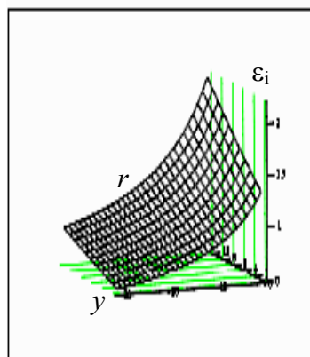
Рис. 4. Распределение интенсивности
