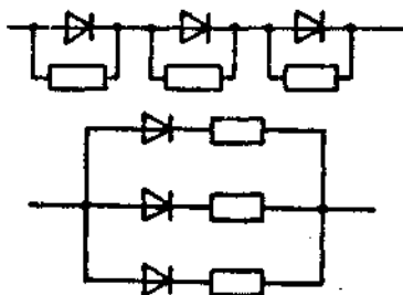
Рис. 2.44. Послідовне і паралельне ввімкнення діодів у радіаційно-стійкій апаратурі
