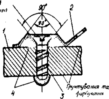
Рис. 2.23. Приєднування пелюстки до литого корпусу самонарізуючими гвинтами: 1 – корпус; 2 – пелюстка; 3 – гвинт; 4 – компаунд ГЗК-6
