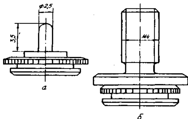
Рис.2.19. Приладові контакти заземлення: а – для круглого монтажної проволу; б - з'єднання проволу з наконечником за допомогою гайки
