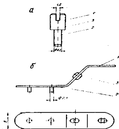
Рис. 2.20. Біметалеві контакти: а – контакти типу "стовпчик"; б – пластинчастий контакт: 1 – мідь, покрита прикусом НОС 61; 2 – алюмінієвий сплав; 3 – місце зварювання
