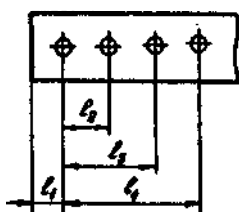
Рис. 3.6. Вибір бази при проставлянні розмірів при штампуванні
