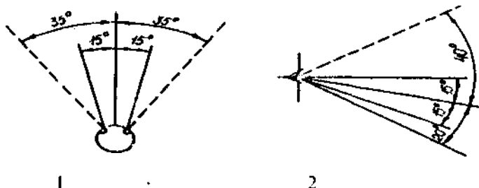
Рис. 2.6. Оптимальні та максимальні кути огляду при повороті очей: 1 - в горизонтальній площині; 2 - у вертикальній площині огляду
