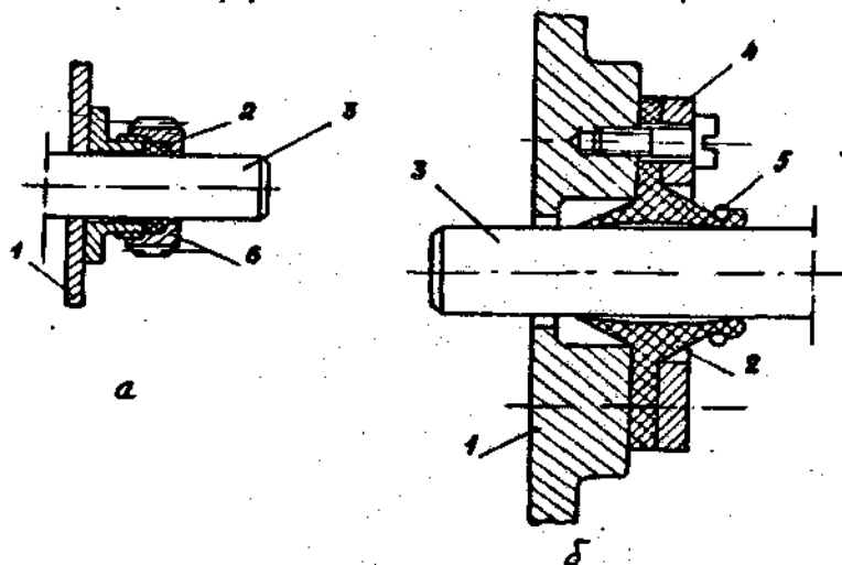
Рис.2.32. Ущільнення валиків герметизованої електронної апаратури за допомогою азбестового (а) і фторопластового (б) сальників: 1 – корпус; 2– сальник; 3– валик; 4– притисний фланець; 5– пружинне кільце; 6– накидна гайка
