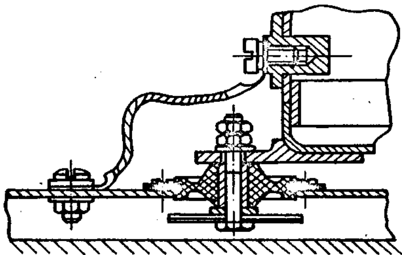
Рис. 2.11. Встановлення блоку на віброізоляторах
