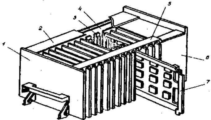
Рис.2.3.Блок рознімної конструкції літакової апаратури:
