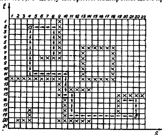
Рис. 4.11. Променевий алгоритм трасування
