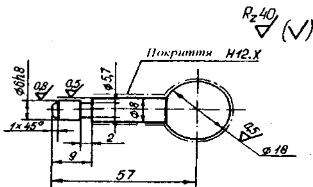
Рис. 2.28. Приклад проставлення на кресленнях позначень покриттів поверхні
