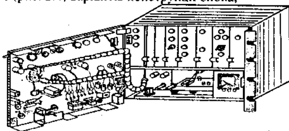
Рис. 2.1. Конструкція блока, що розкривається
