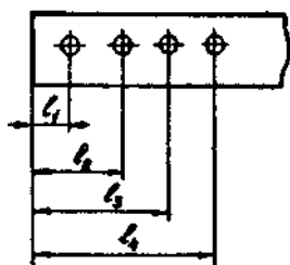
Рис. 3.6. Вибір бази при проставлянні розмірів при штампуванні
