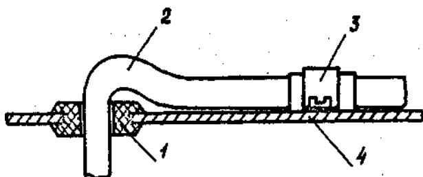
Рис. 3. 36. Приклад прокладки джгута у вікно металевої стінки: 1 - ізоляційна втулка; 2 - джгут; 3 - скоба; 4 - стінка
