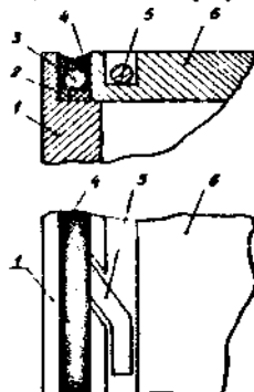
Рис. 2.34. Герметизація корпуса блока мікроелектронної апаратури: 1-корпус; 2-гумова прокладка; 3- лужений дріт; 4- припій; 5- вільний кінець дроту; 6- кришка
