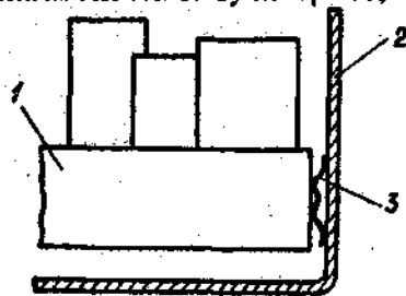
Рис.2.39. Розміщення пластинчастої пружини, яка здійснює тепловий контакт між кожухом і шасі: 1 - шасі; 2 - кожух; 3 - пластинчаста пружина
