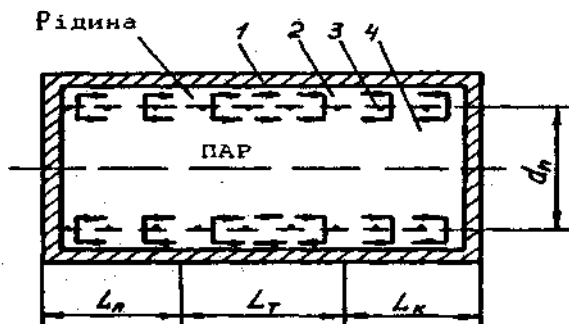
Рис.2.37. Низькотемпературна тепла труба: 1 – герметичний корпус; 2 – гніт; 3 – пружина, що притискує гніт до стінок корпуса; 4 – паровий канал; d_p – діаметр парового каналу; L_v , L_t , L_k – довжина випарної, транспортної та конденсаторної ділянок відповідно
