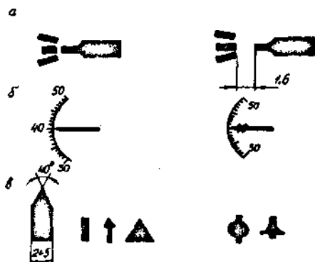
Правильно Неправильно Рис. 3.17. Форма та розміри показників
