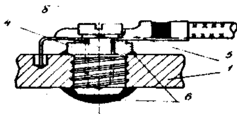
Рис. 2.25. Розрізні затискачі заземлення: а - легкокорозійний затискач; б - затискач під викрутку; 1 - корпус; 2 - гвинт затискача в тілі корпусу; 3 - гайка затискача; 4 - гніздо затискача в тілі корпусу; 5 - гвинт затискача; 6 - компаунд ЕЗК - 6
