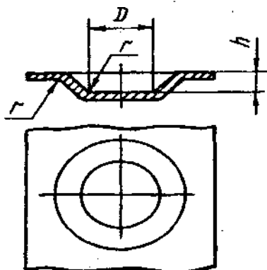
Рис. 3.9. Видавлювання круглої форми
