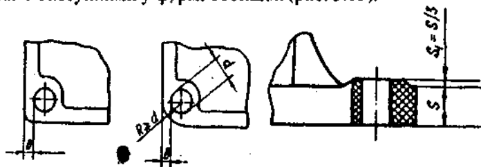
Рис. 3.14. Розташування отвору в куті пластмасової деталі
