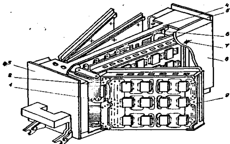
Рис.2.4. Блок книжкової конструкції на мікросхемах і мікроскладаннях: 1 - з'єднувальна колодка; 2 - гнучкий печатний кабель; 3 - передня панель блока; 4 - рама; 5 - задня панель; 6 - з'єднувальна печатна плата; 7 - стяжний гвинт; 8 - бокова стінка; 9 - чарунка
