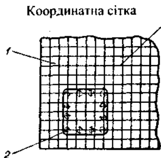
Рис. 3.28. Розміщення корпусних мікросхем зі штирковими виводами (2) на печатній платі зі стандартною координатною сіткою (1) (крок виводів не кратний 2,50 мм)
