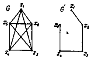
Повний граф
