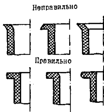
Рис.3.12. Зміцнювальні буртики для тонкостінних деталей
