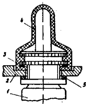
Рис. 2.33. Ущільнення рукоятки тумблера за допомогою ковначка: 1- тумблер; 2- лицьова панель; 3- металева шайба; 4- ковначок; 5- гумова прокладка
