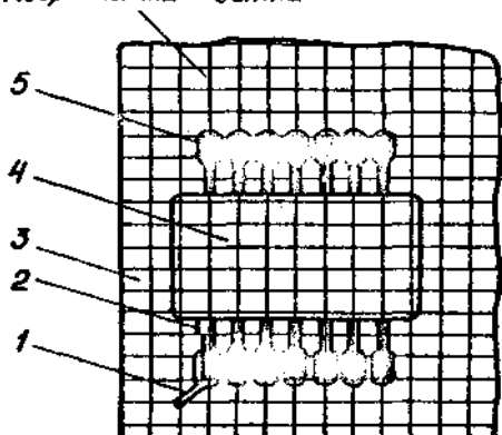
Рис. 3.29. Розміщення корпусних мікросхем з планарними виводами на печатній платі зі стандартною координатною сіткою: 1 – ключ; 2 – перший вивід корпусу ІС; 3 – печатна плата; 4 – корпус ІС; 5 – контактна площадка
