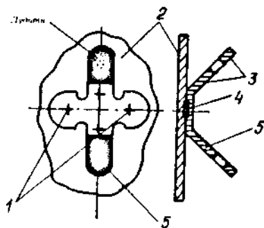
Рис. 2.22. Контактна пелюстка з плакованого алюмінію, що з'єднується з корпусом з листового алюмінієвого сплаву точковим контактним електрозварюванням: 1 – місце зварювання; 2 – корпус; 3 – дужена ділянка пелюстки; 4 – плакований шар міді; 5 – пелюстка
