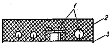
Рис. 2.8. Печатний вузол, залитий з боку радіоелементів вібропоглинальним пінополіуретаном: 1 - радіоелементи; 2 - пінополіуретан; 3 - плата
