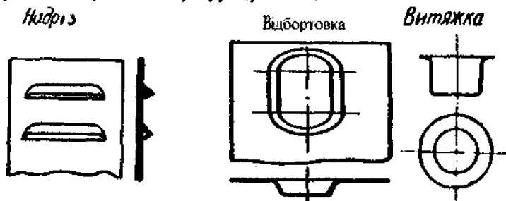
Рис. 3.2. Одержання жалюзі в корпусах електронної апаратури
