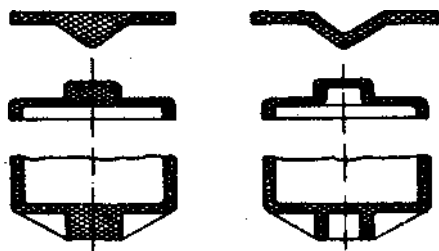
Рис. 3.11. Забезпечення рівності стінки
