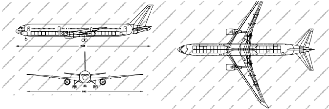
Рисунок 1.4 - Схема літака Boeing 767-400ER
