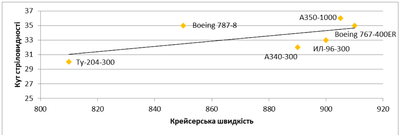
Рисунок 1.9 - Графік залежності стрілоподібності крила від крейсерської швидкості літака
