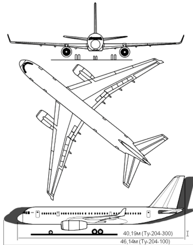
Рисунок 1.5 - Схема літака Ту-204-300
