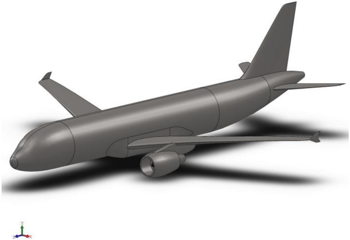
Рисунок 1.14 Майстер-геометрія проєктованого літака
