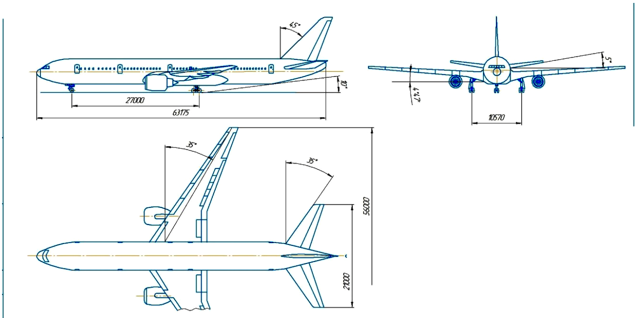
Рисунок 1.12 Схема літака
