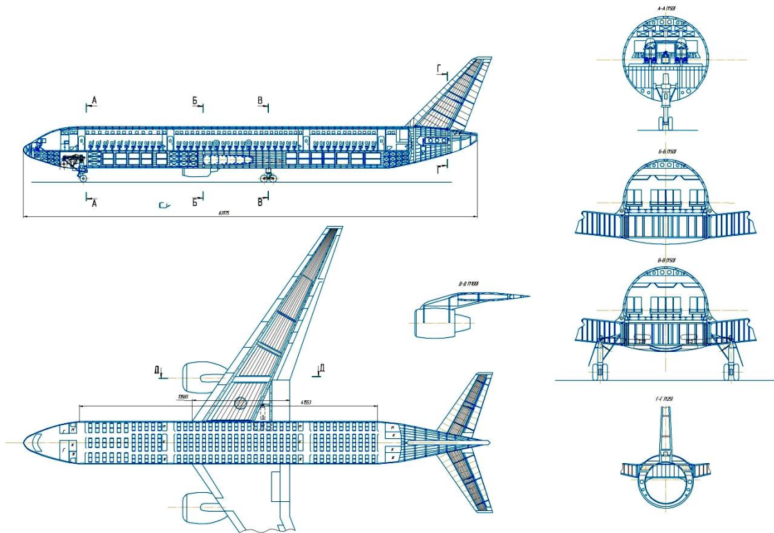
Рисунок 1.13 Компонівка літака
