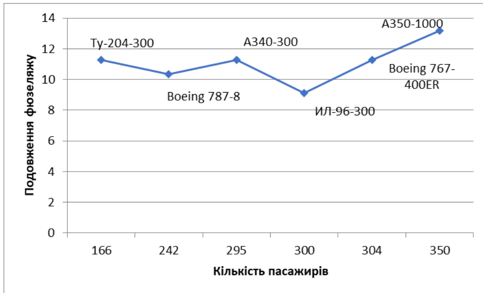
Рисунок 1.10 - Графік залежності подовження фюзеляжу від кількості пасажирів
