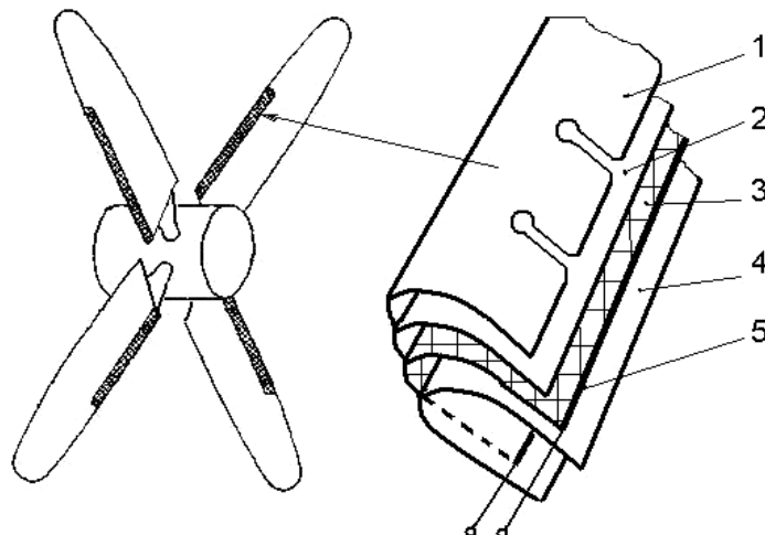
Fig. 4.12. Heating element:
