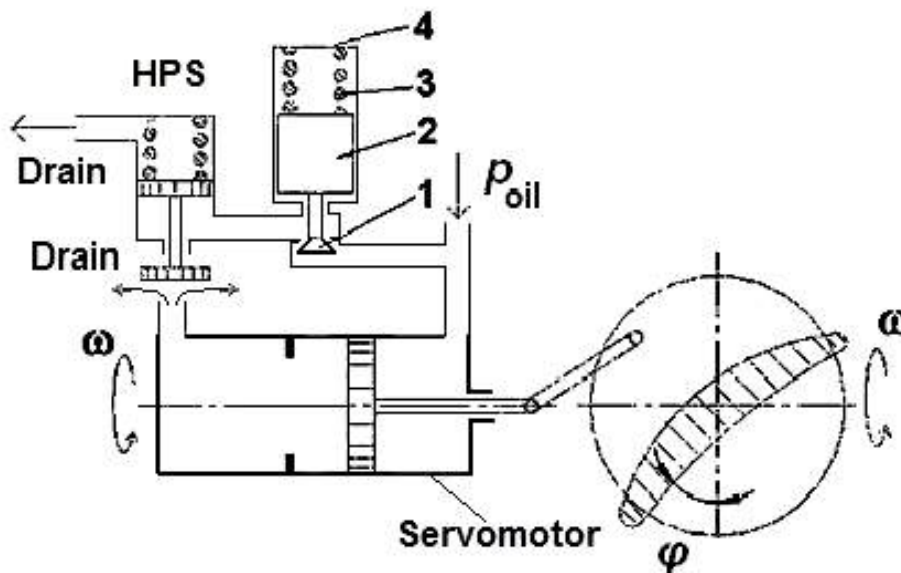
Fig. 3.4. Centrifugal pitch stop:
