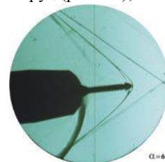
Рис. 12. Візуалізація картини надзвукового обтікання
