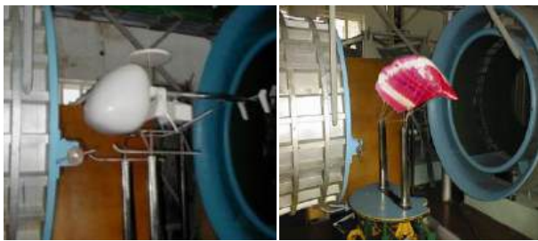
Рис. 5. Аеродинамічна труба дозвукових швидкостей Т-4
