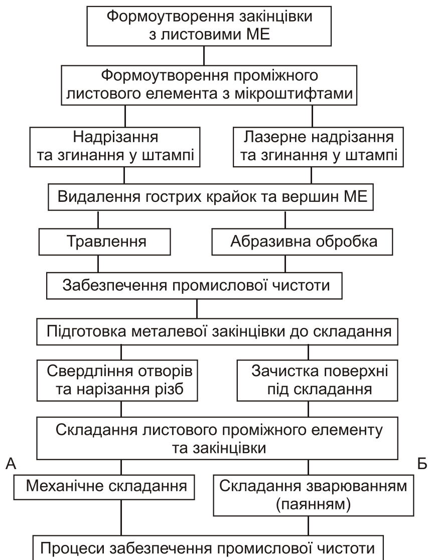
Рис. 3. Варіанти маршрутних техпроцесів формоутворення трансверсальних зв'язків на металевих закінцівках з використанням листових підсилювальних елементів
