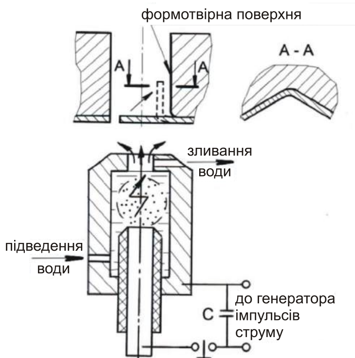
Рис. 5. Схема електрогідравлічного пристрою для згинання надрізаних ділянок на кут 90^\circ імпульсним струменем рідини з формоутворенням неплаского перерізу відігнутої ділянки
