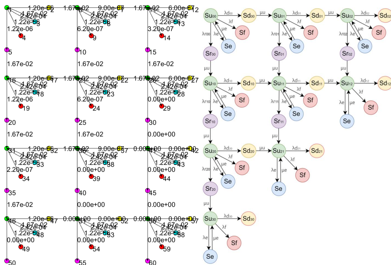
Рисунок 3.27 – МФМЗ з БРД та реконфігурацією в Matlab та draw.io
