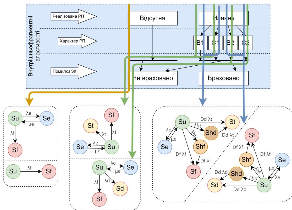
Рисунок 3.6 – Формування множин типових ОФМ
