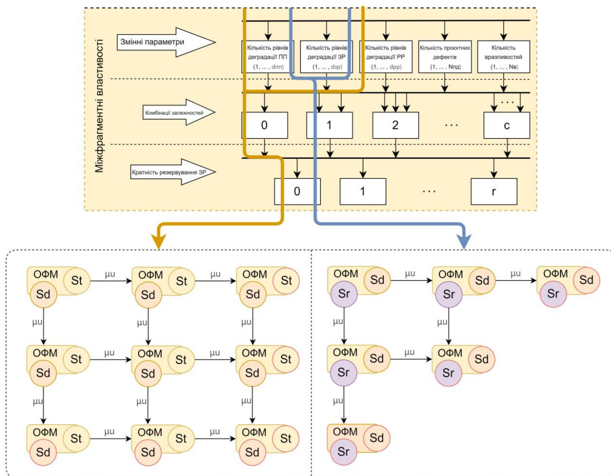
Рисунок 3.8 – Формування множин двовимірних МФМ (прямокутнікова/трикутнікова)
