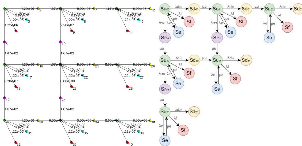
Рисунок – 3.23 МФМ2 з БРД та реконфігурацією в Matlab та draw.io
