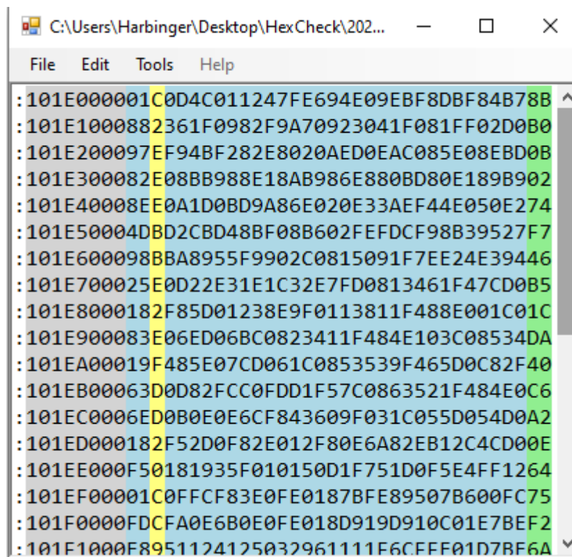
Рисунок 4.8 – Візуалізація коригування даних у “FixAVRHexChecksum”
