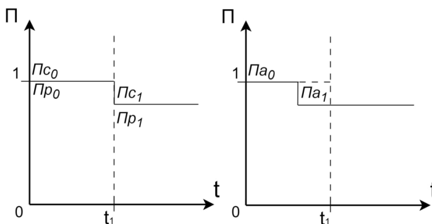
Рисунок 2.15 – Різниця впливу ЗР між Пр та Па деградаціями
