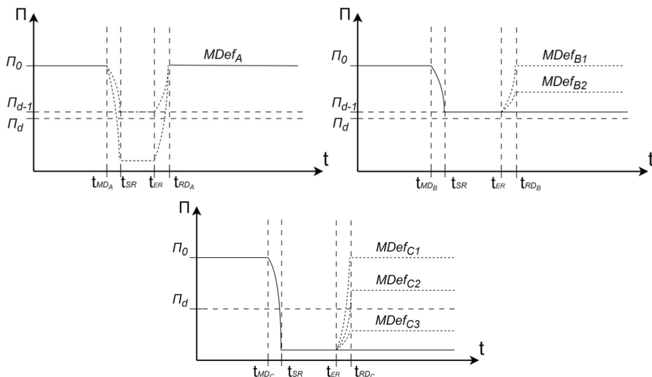
Рисунок 2.1-3 – Діаграми деградації прояву розглянутих множин дефектів
