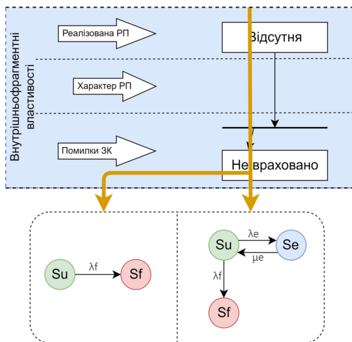
Рисунок 3.3 – Формування множин ОФМ без потенційної реконфігуроприсадаєтності
