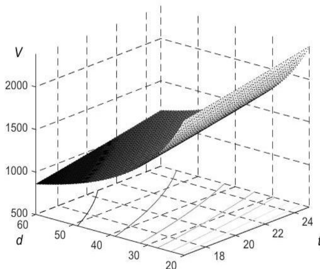
Рис. 4.1 Поверхня залежності потреби в обсягах води на зрошення від середньомісячної температури повітря та кількості опадів у степовій зоні протягом вегетаційного періоду [за авторськими розрахунками]
