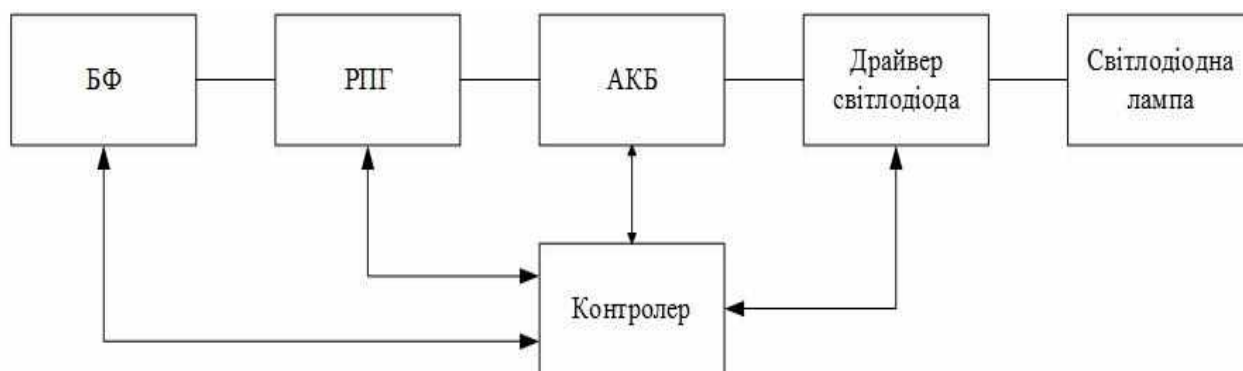
Рис. 1. Система електроживлення автономної сонячної системи вуличного освітлення (БФ – батарея фотоелектрична, РПГ – регулятор потужностей генератора, АКБ – акумуляторна батарея)
