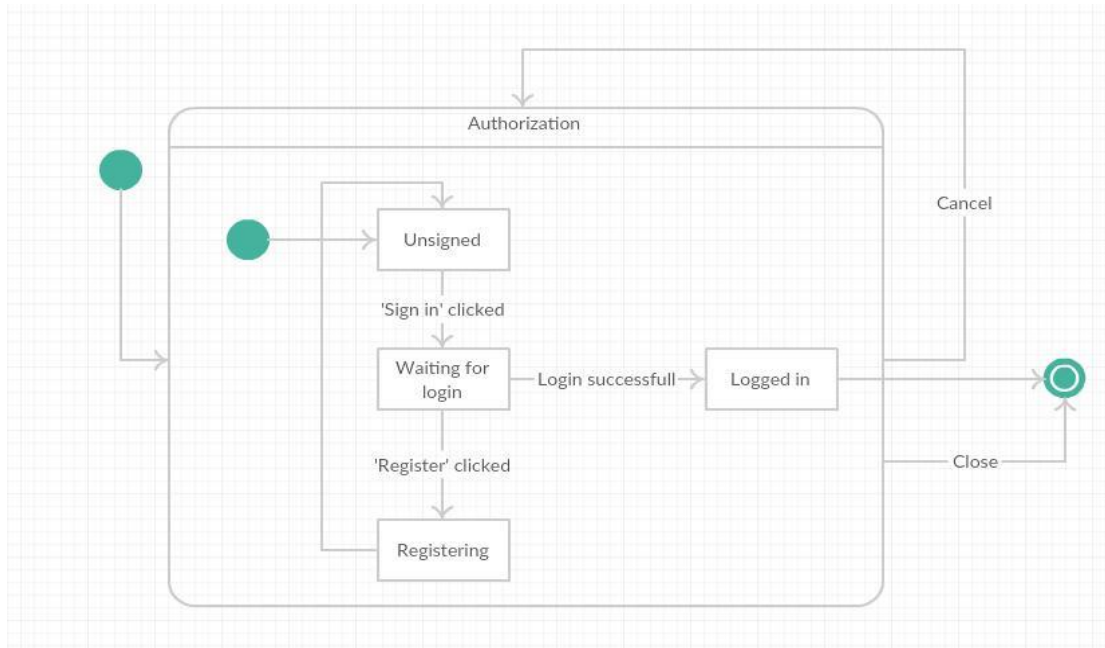
Рисунок 3.5 – Діаграма станів
