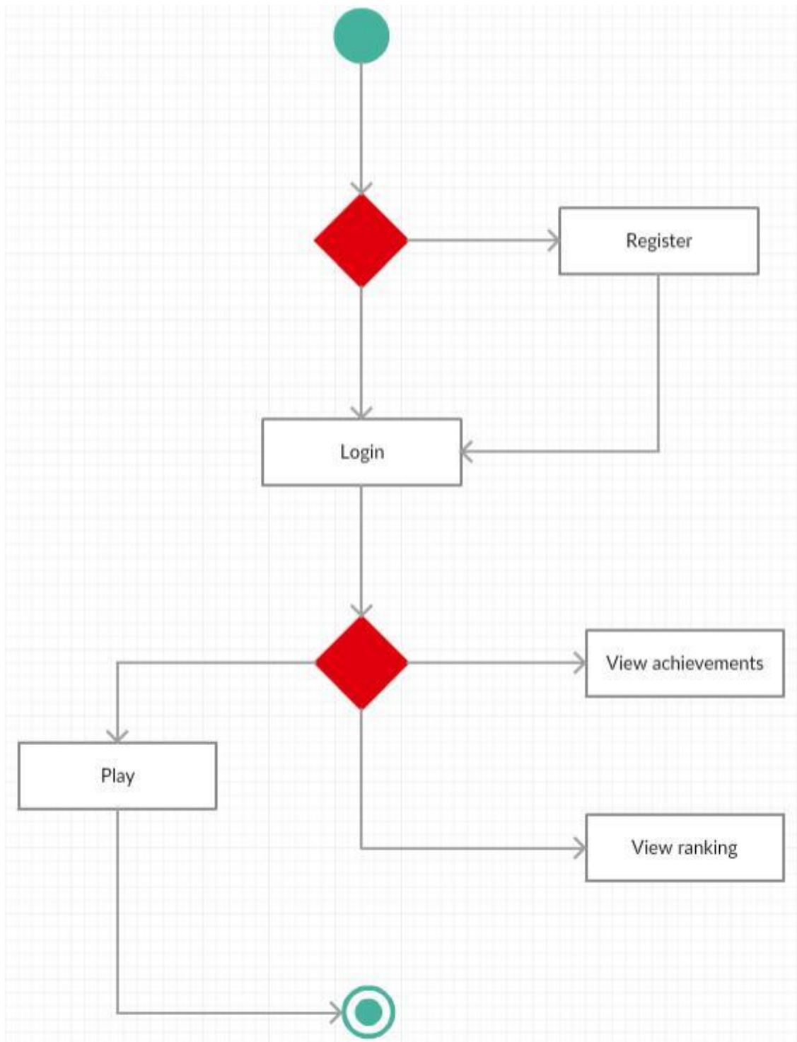
Рисунок 3.4 – Діаграма діяльності
