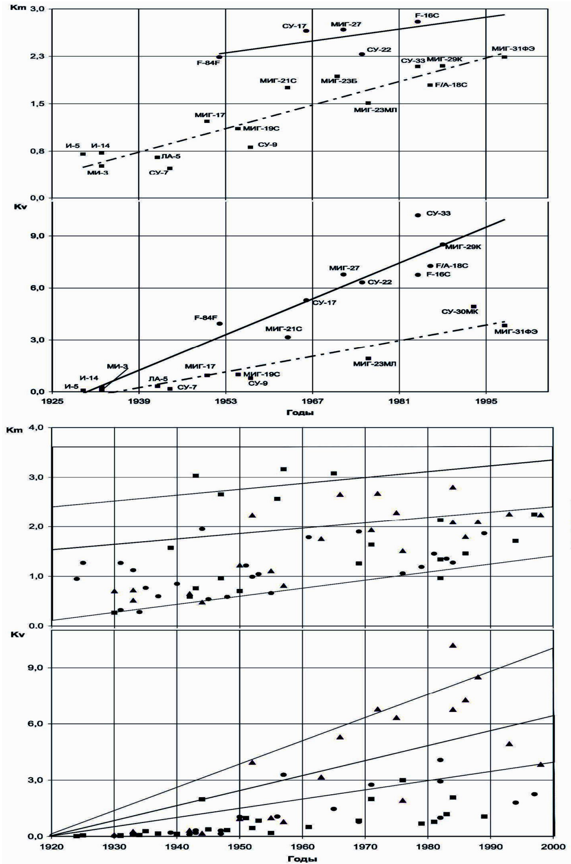
Рис. 1. Развитие массового и скоростного совершенства аэродинамических транспортных систем: Б (■) – бомбардировщики, И (▲) – истребители, Т (●) – транспортные самолеты
