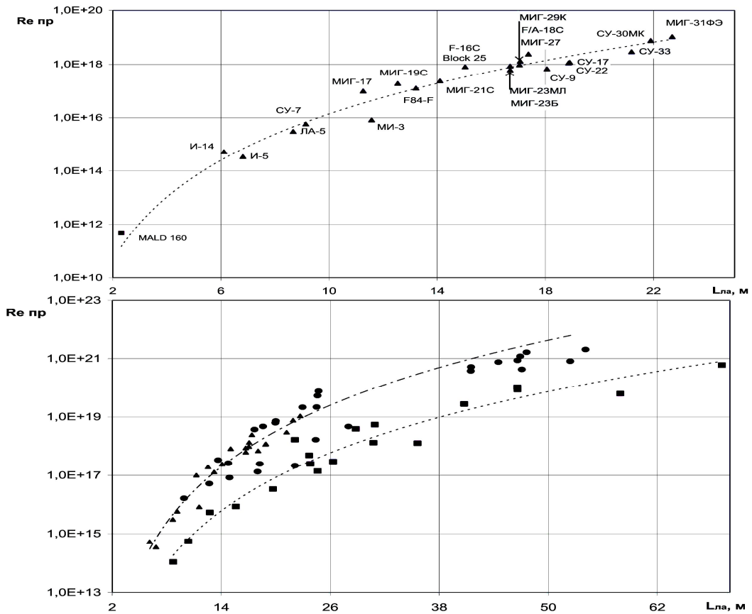
Рис. 3. Изменение приведенного числа Рейнольдса в зависимости от размера летательного аппарата
