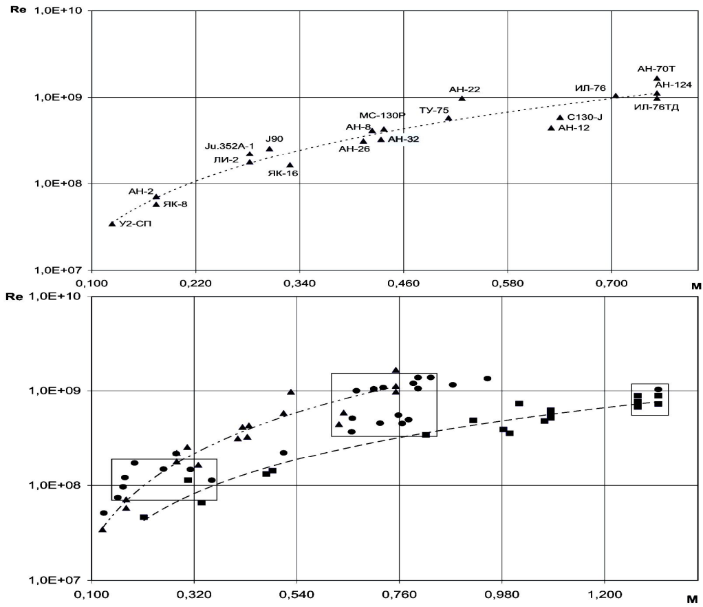
Рис. 2. Изменение числа Re в зависимости от M полета (---- – max; - - - - – min)
