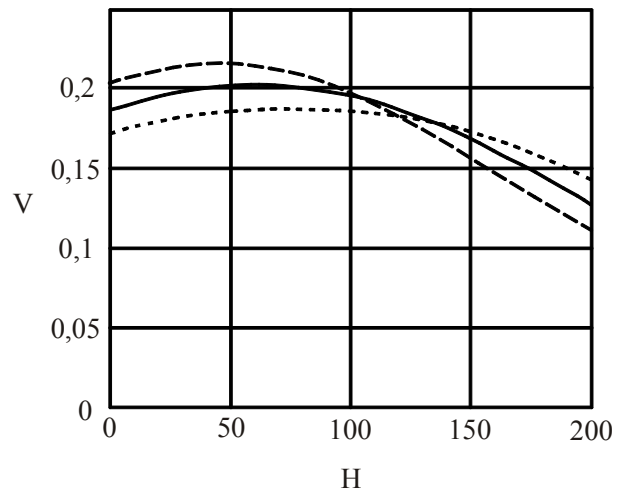
Рис. 8. Зависимость скорости нанесения покрытия по высоте обрабатываемой детали: - - - - при l = 90 мм; — при l = 120 мм; ..... при l = 150 мм.
