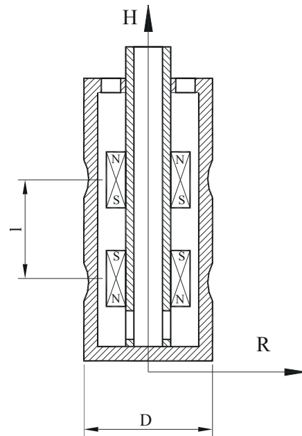
Рис. 7. Использование двух зон распыления
