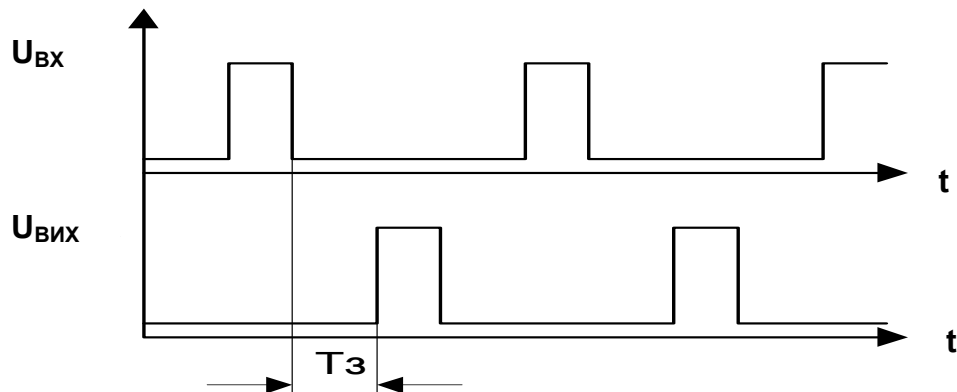
Рис. 4.13. Затримка відеоімпульсів
