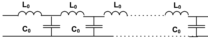
Рис. 4.15. Еквівалентна схема однорідної лінії затримки
