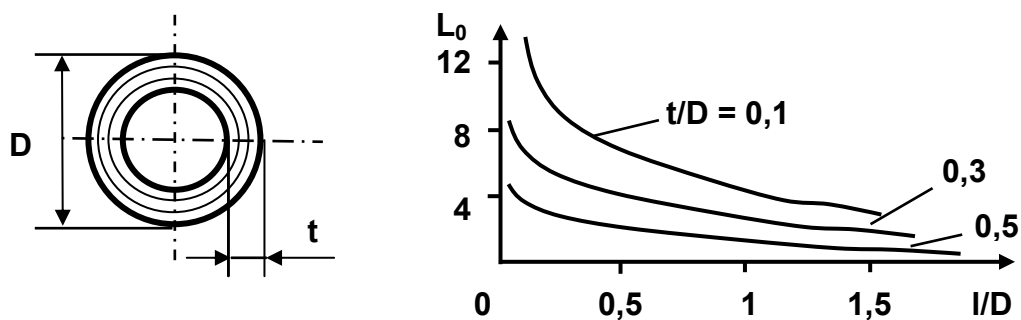
Рис. 4.4. Поправковий коефіцієнт для багатошарової котушки
