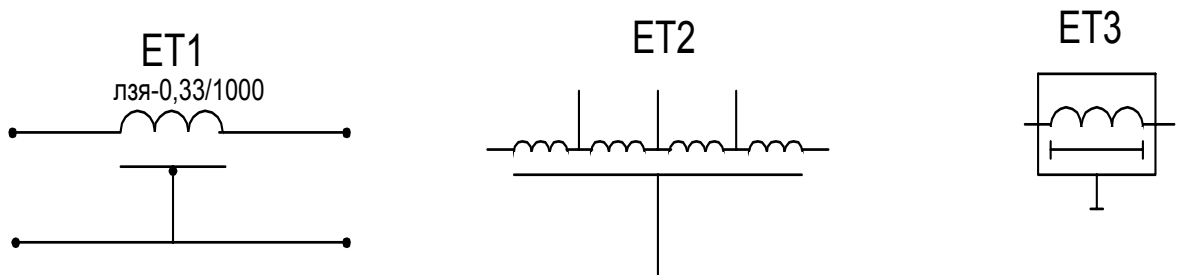
Рис. 4.14. Позначення ліній затримки на схемах
