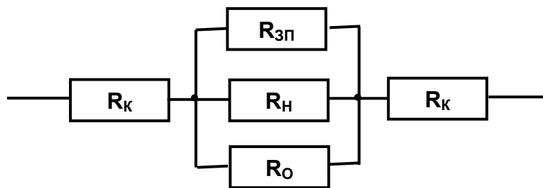
Рис. 2.14. Схема заміщення резистора на постійному струмі
