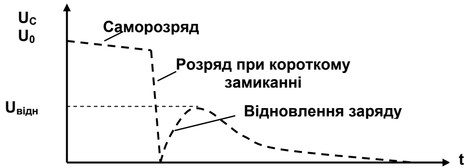
Рис. 3.10. Зміна заряду на конденсаторі при абсорбції
