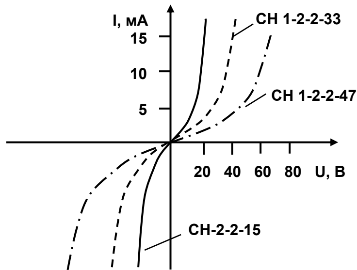
Рис. 2.6. Вольт-амперні характеристики варисторів
