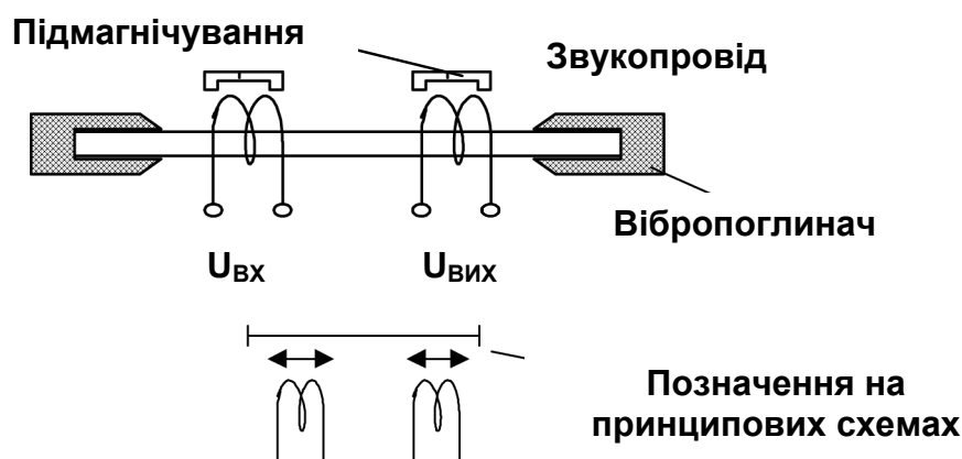
Рис. 4.20. Магнітострикційні ЛЗ
