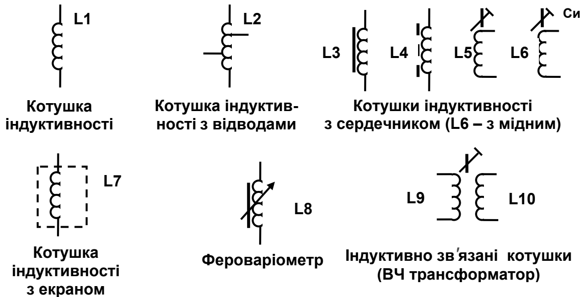
Рис. 4.1. Позначення котушок індуктивності на схемах
