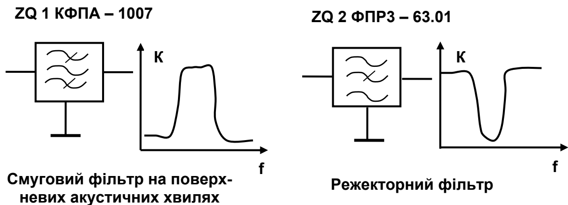
Рис. 4.9. Позначення й частотні характеристики ПКФ фільтрів
