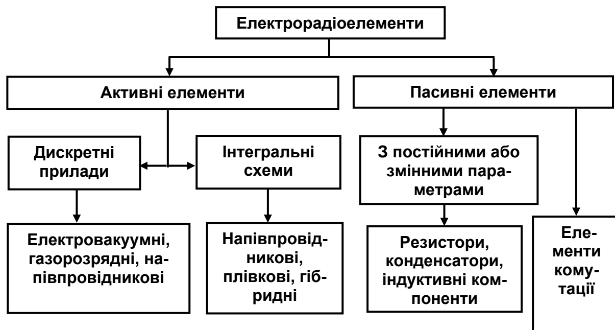
Рис. 1.1. Класифікація електрорадіоелементів
