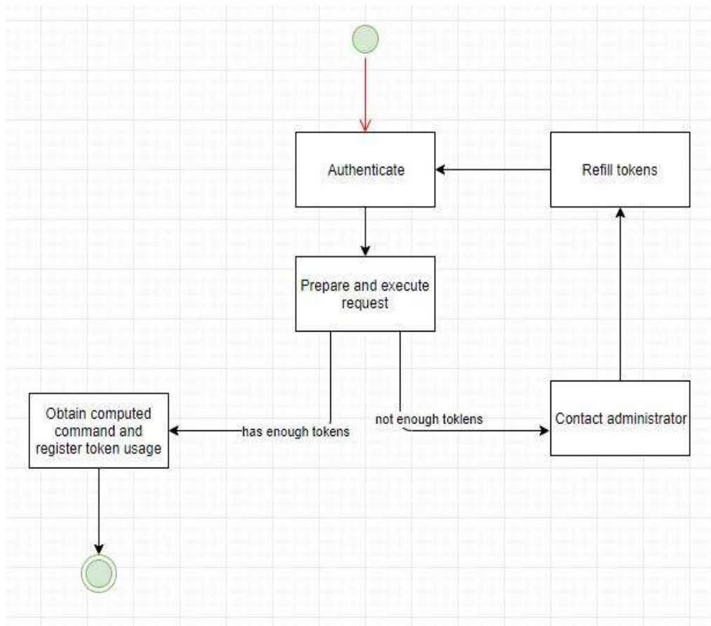
Рисунок 3.5 – Діаграма станів
