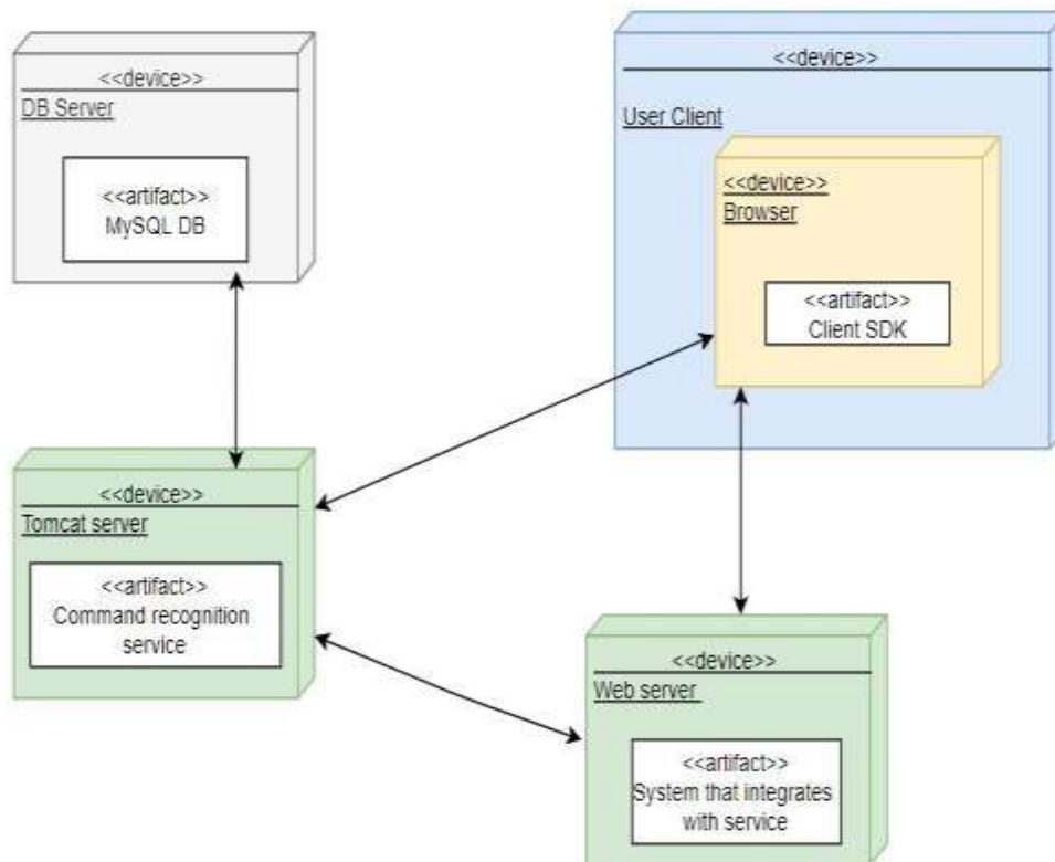
Рисунок 3.6 – Діаграма розгортання
