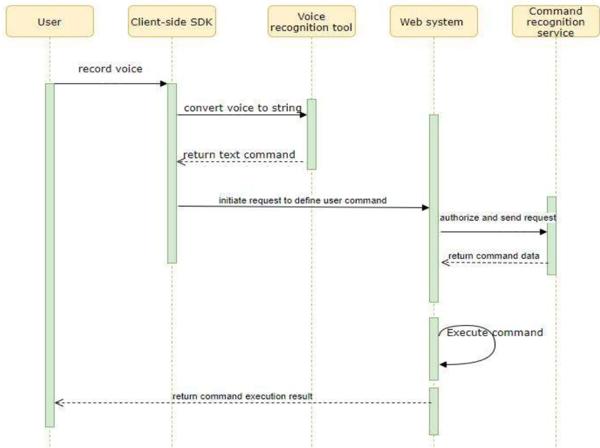
Рисунок 3.4 – Діаграма послідовностей
